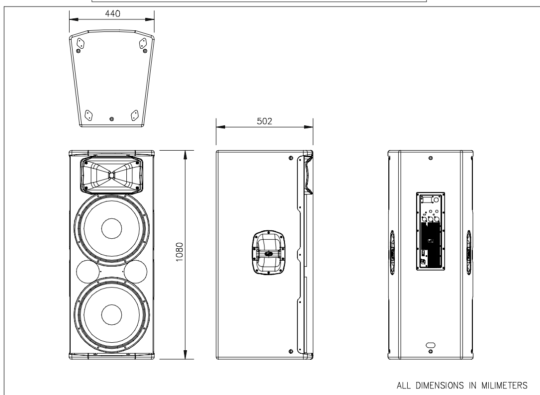
vantec 215A
